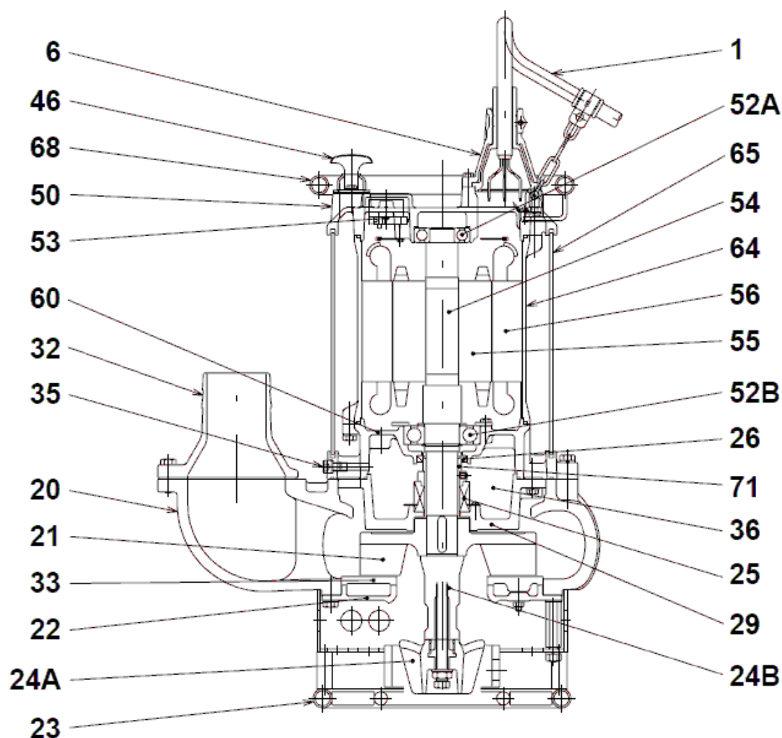
GPN3-100
