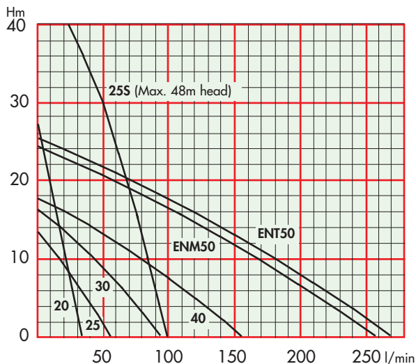
TYPE 20
